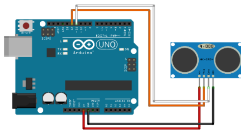
Рис. 2.3.6. Схема подключения ультразвукового датчика.
