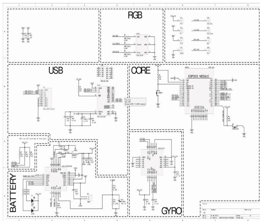
Рисунок 7. Схема трекера системы захвата движения «PROMETHEY»
