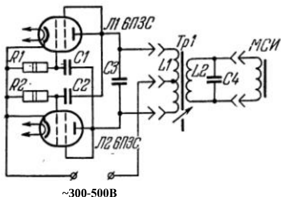
Рисунок 2. Электрическая схема лампового ультразвукового генератора и готовая модель
