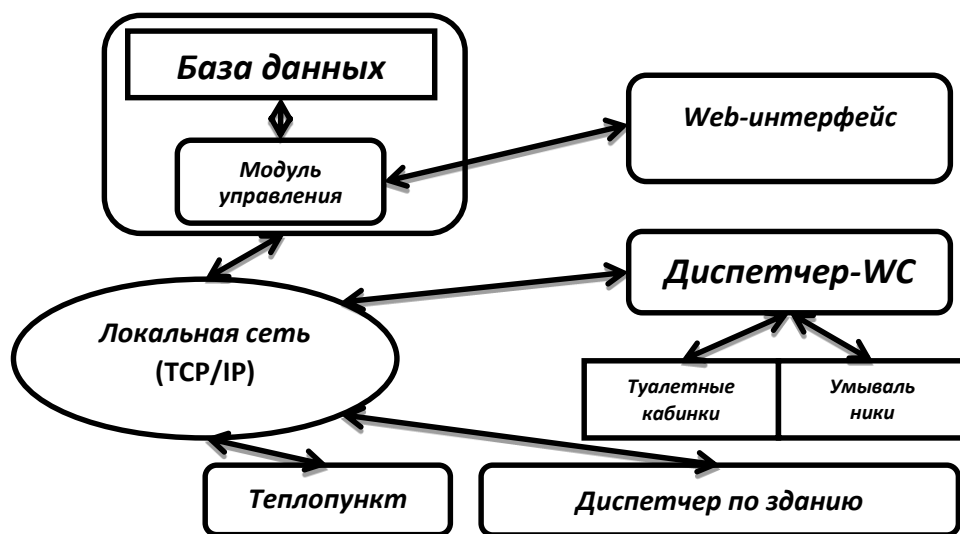
Рисунок 1. Схема работы системы
