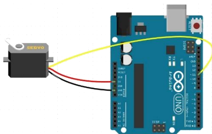
Рис. 2.3.12. Схема подключения микросервопривода.
