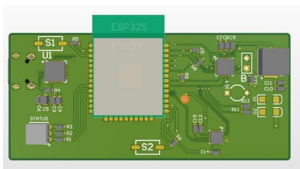
Рисунок 8. Рендер платы, вид сверху
