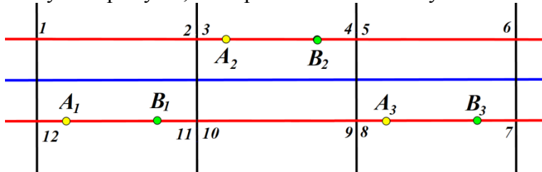
Рисунок 5. Орбита прямой 2
